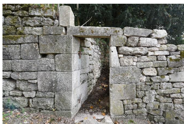
État du mur après restauration (octobre 2021)
